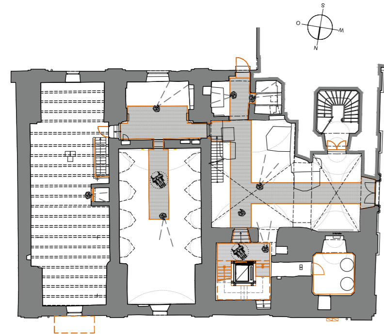
Grundriss Erdgeschoß
