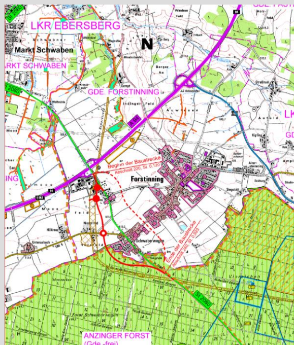
St 2080 Markt Schwaben – Ebersberg Ortsumfahrung Schwaberwegen
